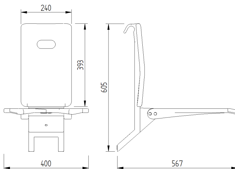
Technische Zeichnung
