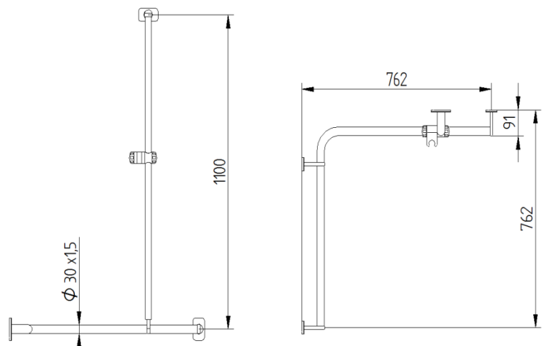
Technische Zeichnung (Ausführung Rechts)
