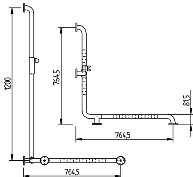
Technische Zeichnung (Ausführung Rechts)
