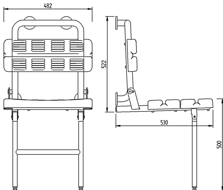
Technische Zeichnung
