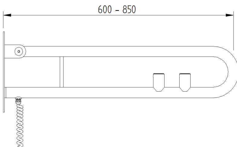
Technische Zeichnung
