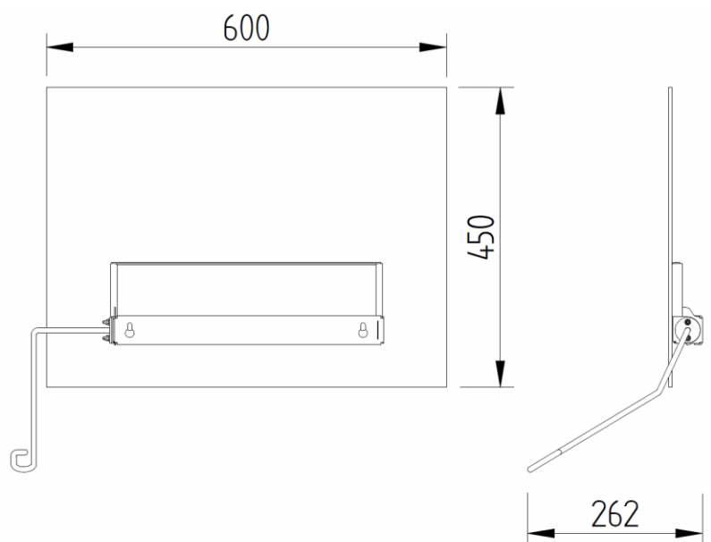
Technische Zeichnung (Ausführung Rechts)
